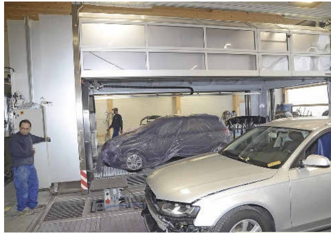
Bei geöffneten seitlichen Rolltoren kann die Kabine verschoben werden – je nach gewählter Option von Hand oder elektrisch.
